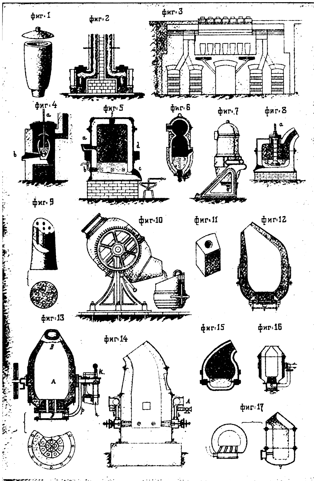
1. Тигель для плавки стали; фиг. 2. Тигельный горн; фиг. 3. Регенеративная печь для тигельной стали; фиг. 6, 7, 8, 10 и 15. Разные формы реторты Бессемера; фиг. 9. Фурма; фиг. 11. Фурменный кирпич; фиг. 12. Реторта с дномъ Holley; фиг. 13. Реторта сь кирпичнымъ дномъ; фиг. 14, 16 и 17. Реторты для малыхъ насадокъ.
